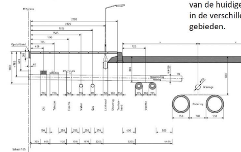
B.4 Voorbeeld dwarsprofiel voor een woonstraat
